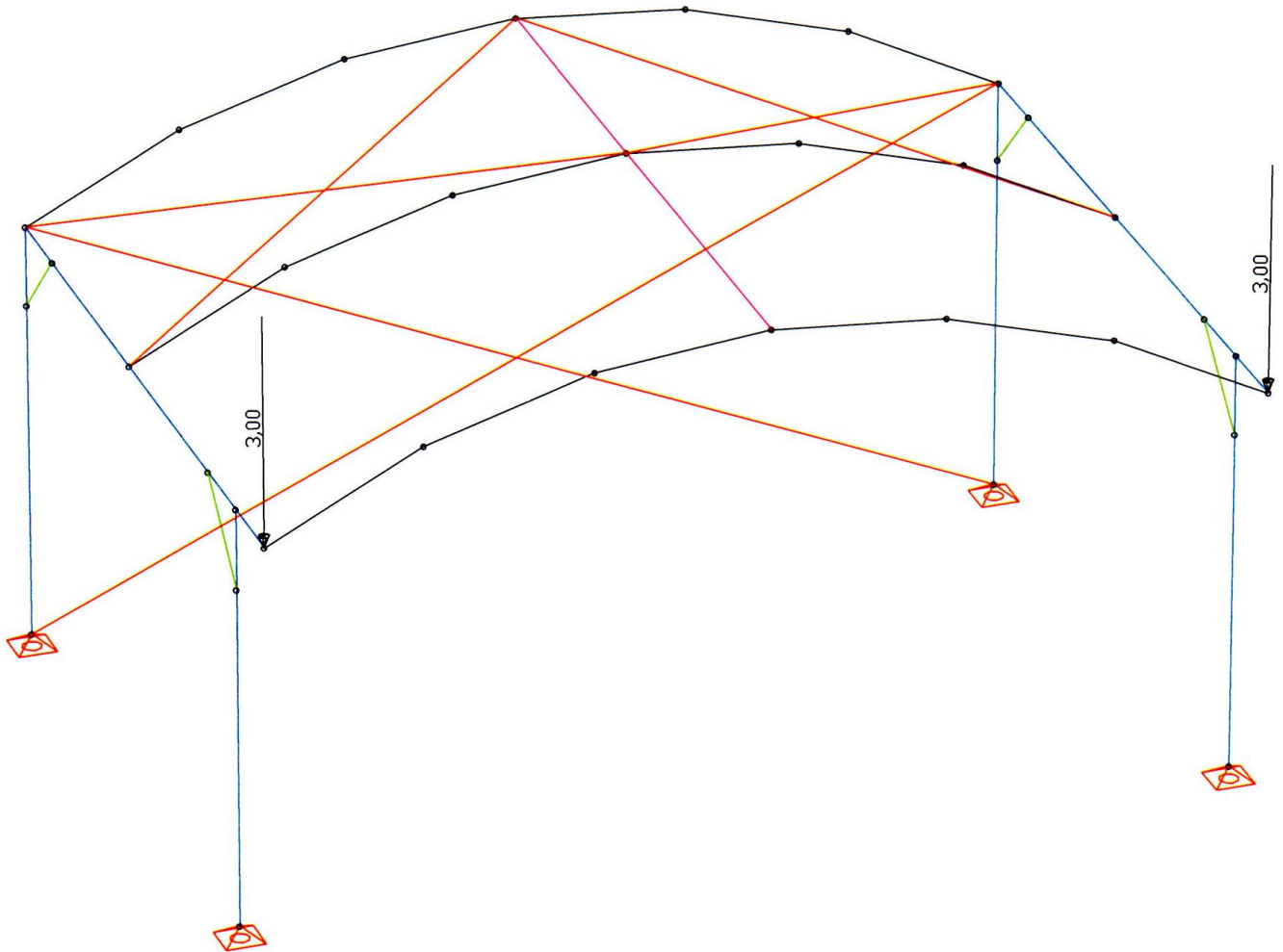
LF 5: Belastung, PA-load
